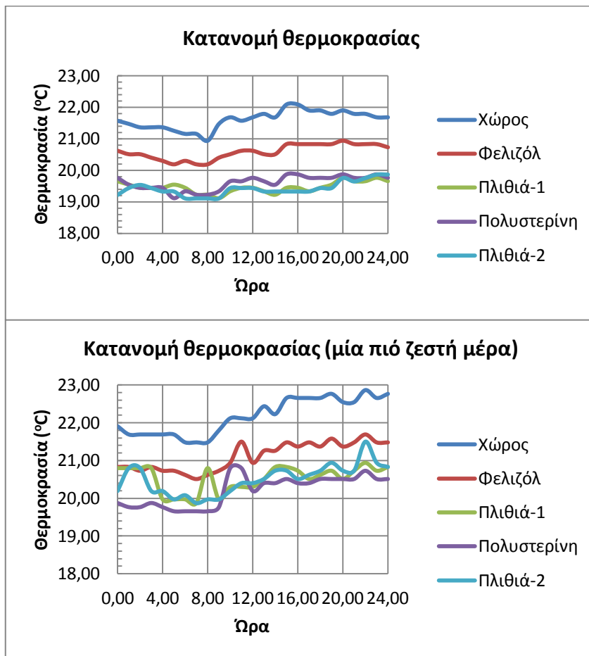
Σχήμα 8 : Κατανομή θερμοκρασίας δύο διαφορετικές ημέρες
