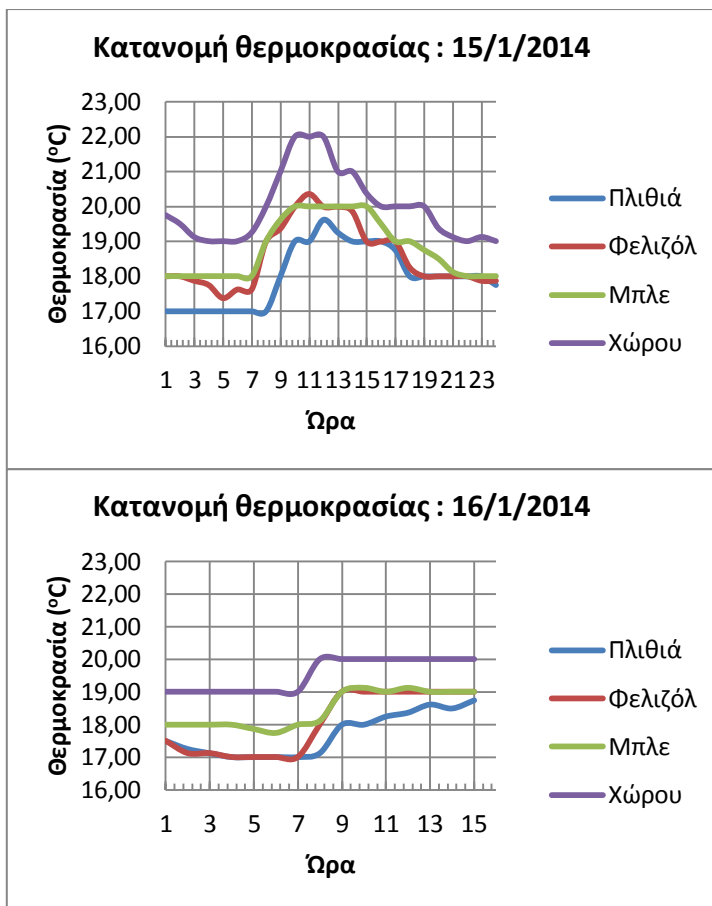
Σχήμα 10 : Κατανομή θερμοκρασιών στα 3 "σπίτια"
