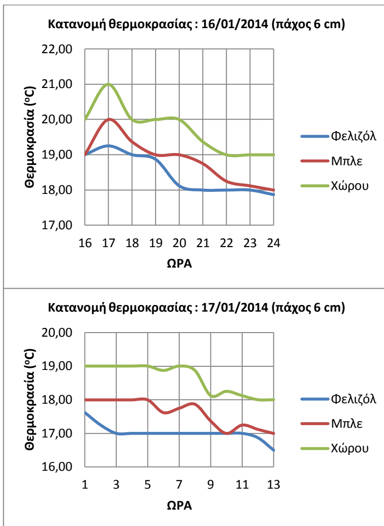
Σχήμα 11 : Κατανομή θερμοκρασιών στα σπίτια από πολυστερίνη πάχους 6cm
